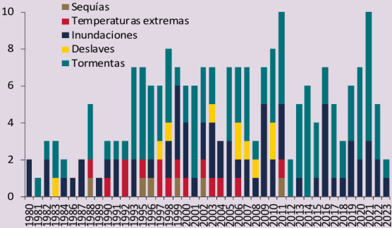
Gráfica 2 Frecuencia de desastres relacionados con el clima en México por tipo de desastre Número de desastres
