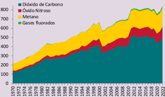
Gráfica 1 Emisiones de gases de efecto invernadero (GEI) en México por tipo de gas MtCO 2 e
