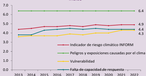
Gráfica 3 Desglose del Índice de riesgo climático global INFORM para México Índice
